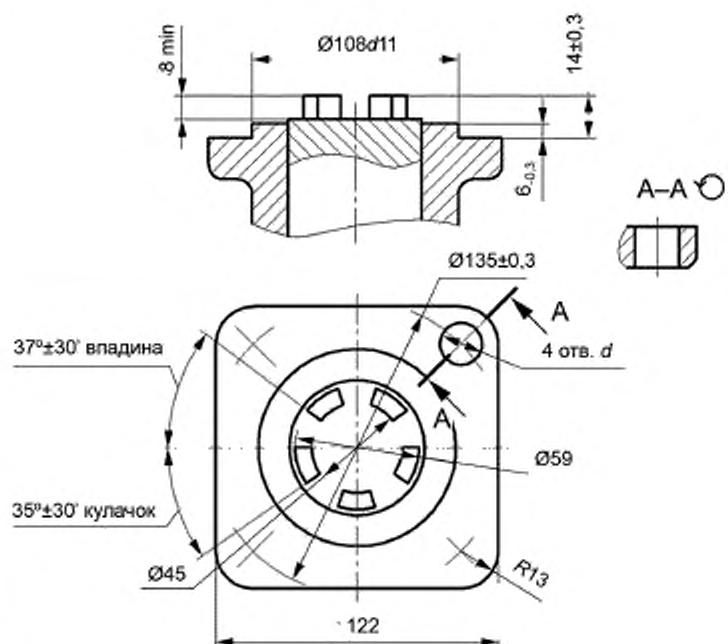
Рисунок А.10 — Ответное присоединение трубопроводной арматуры типа Б
