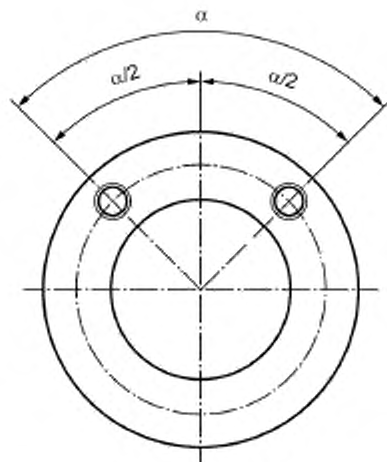
Рисунок 3 — Расположение отверстий для типов присоединений F03—F100
