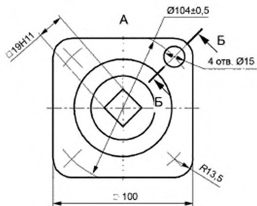
Рисунок А.5 — Присоединение привода типа АЧ
