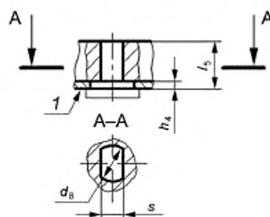
Рисунок 18 — Соединения с лысками
