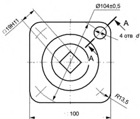
Рисунок А.6 — Ответное присоединение трубопроводной арматуры типа АЧ
